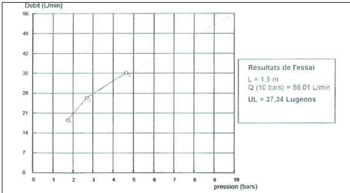
Figure : courbe d'essai Lugeons du sondage 3
