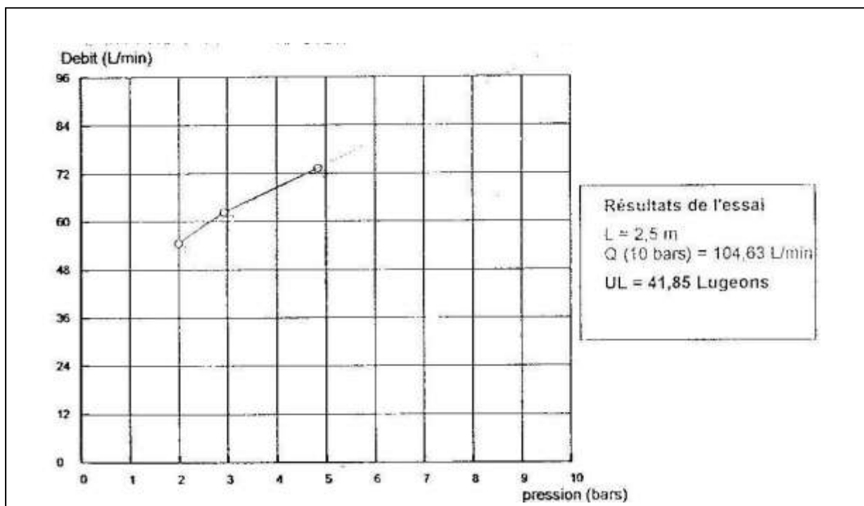
Figure : courbe d'essai Lugeons du sondage 2
