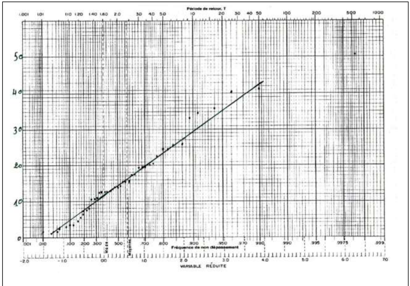
Figure II.10 : Ajustement de la loi de Gumbel à l'échantillon des P_{J \max} observés à Tamanrasset.
