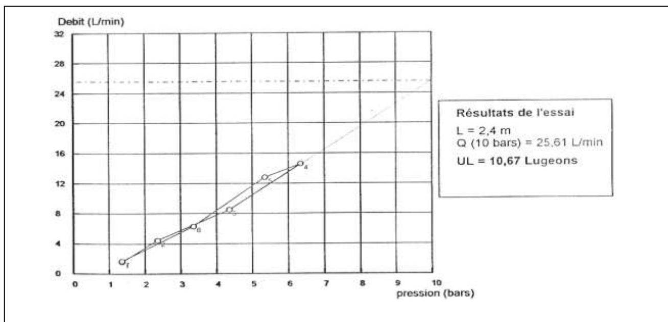
Figure : courbe d'essai Lugeons du sondage 9
