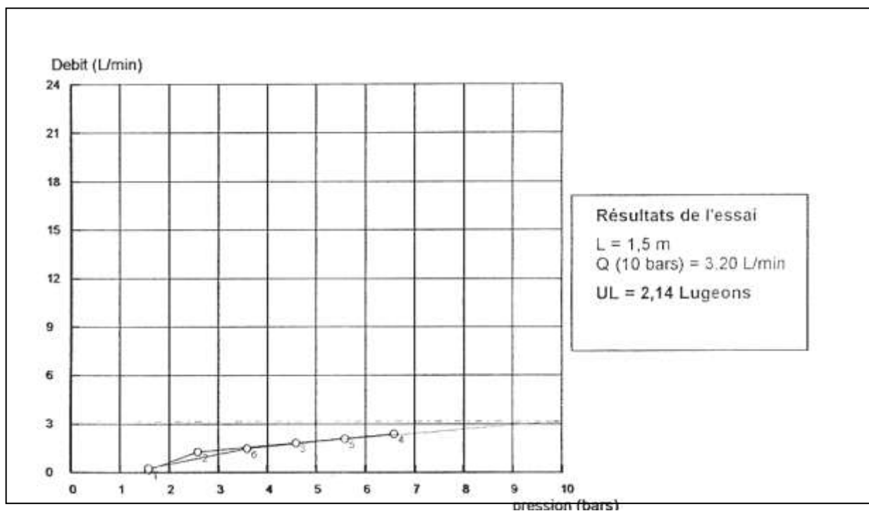
Figure : courbe d'essai Lugeons du sondage 8
