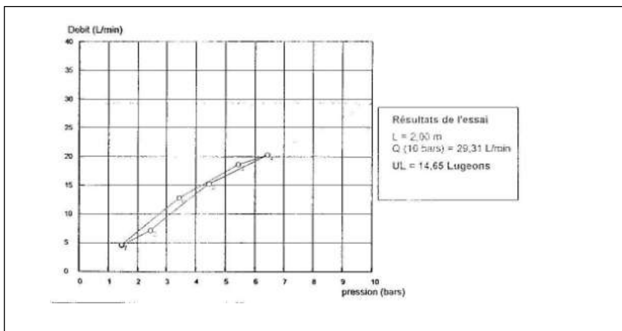
Figure : courbe d'essai Lugeons du sondage 6
