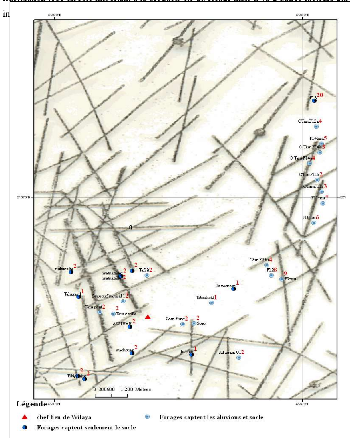
Figure I.16 : carte de fracturation et point d'eaux de la zone d'étude
