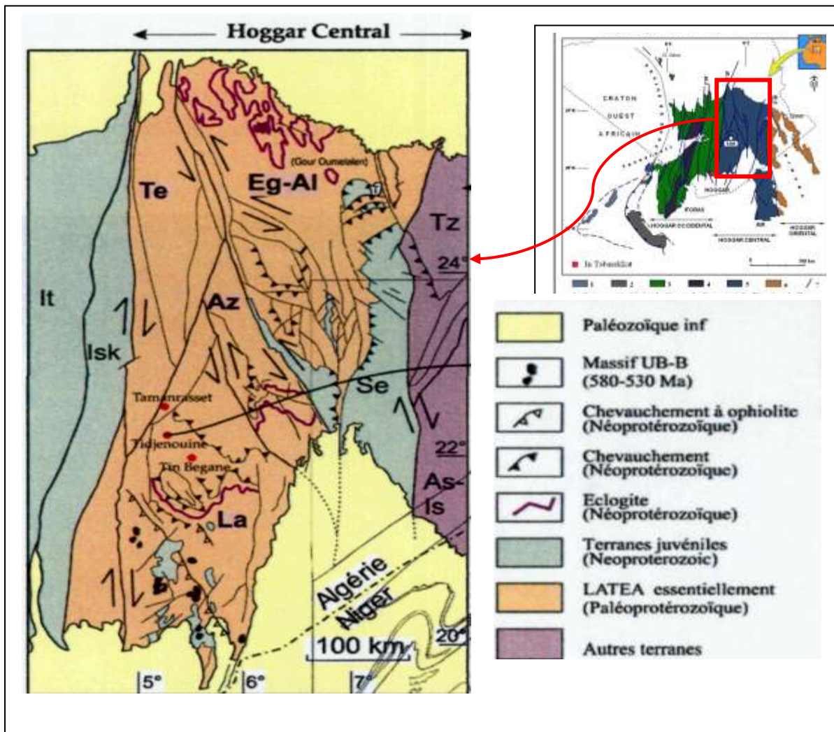
Figure I.7 : le Hoggar central (Léigeois et al, 2003)
