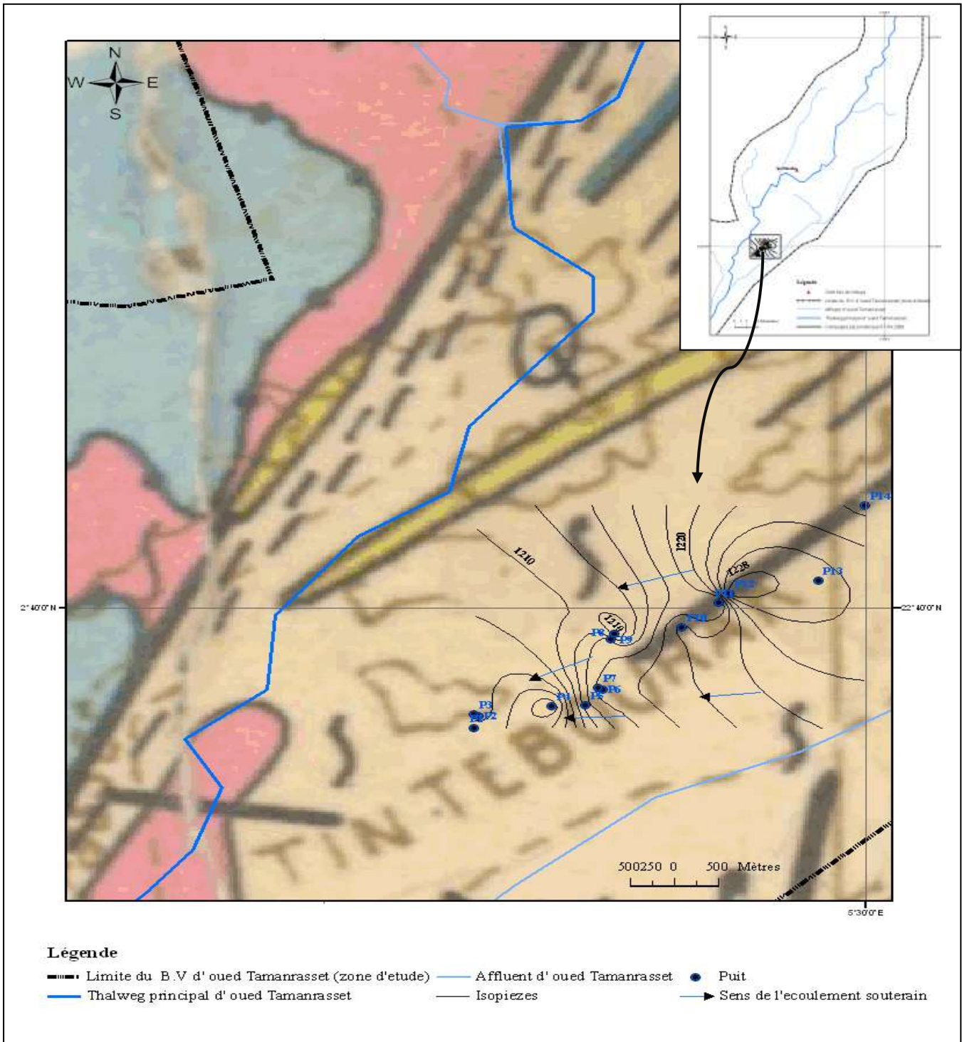
Figure III.10 : Carte piézométrique 01-04-2008 (Amsel).
