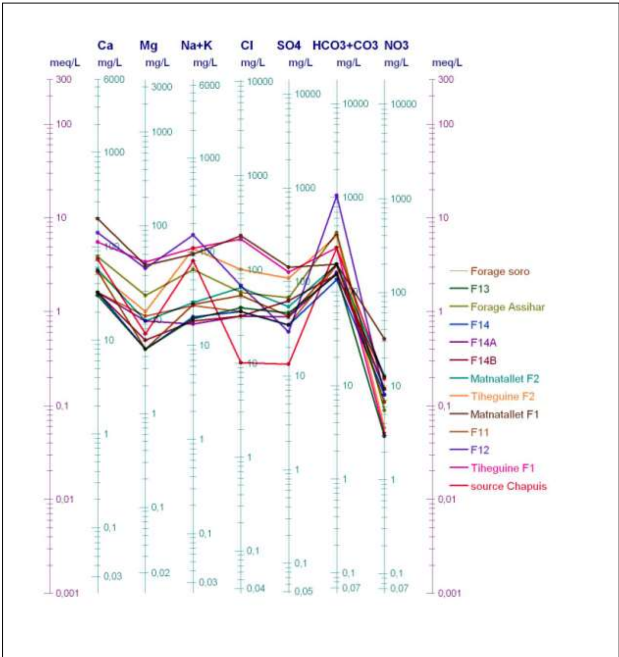
Figure IV.4 : diagramme Shoeller-Berkalof des eaux.
