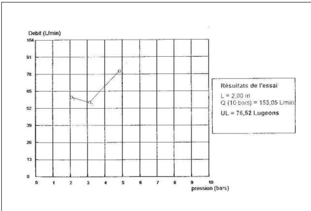
Figure : courbe d'essai Lugeons du sondage 1 (tranche 14.00-16.00)
