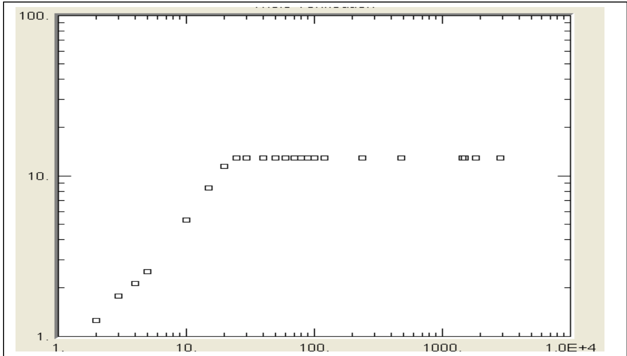
Figure III.19 : courbe de descente du forage Machouen
