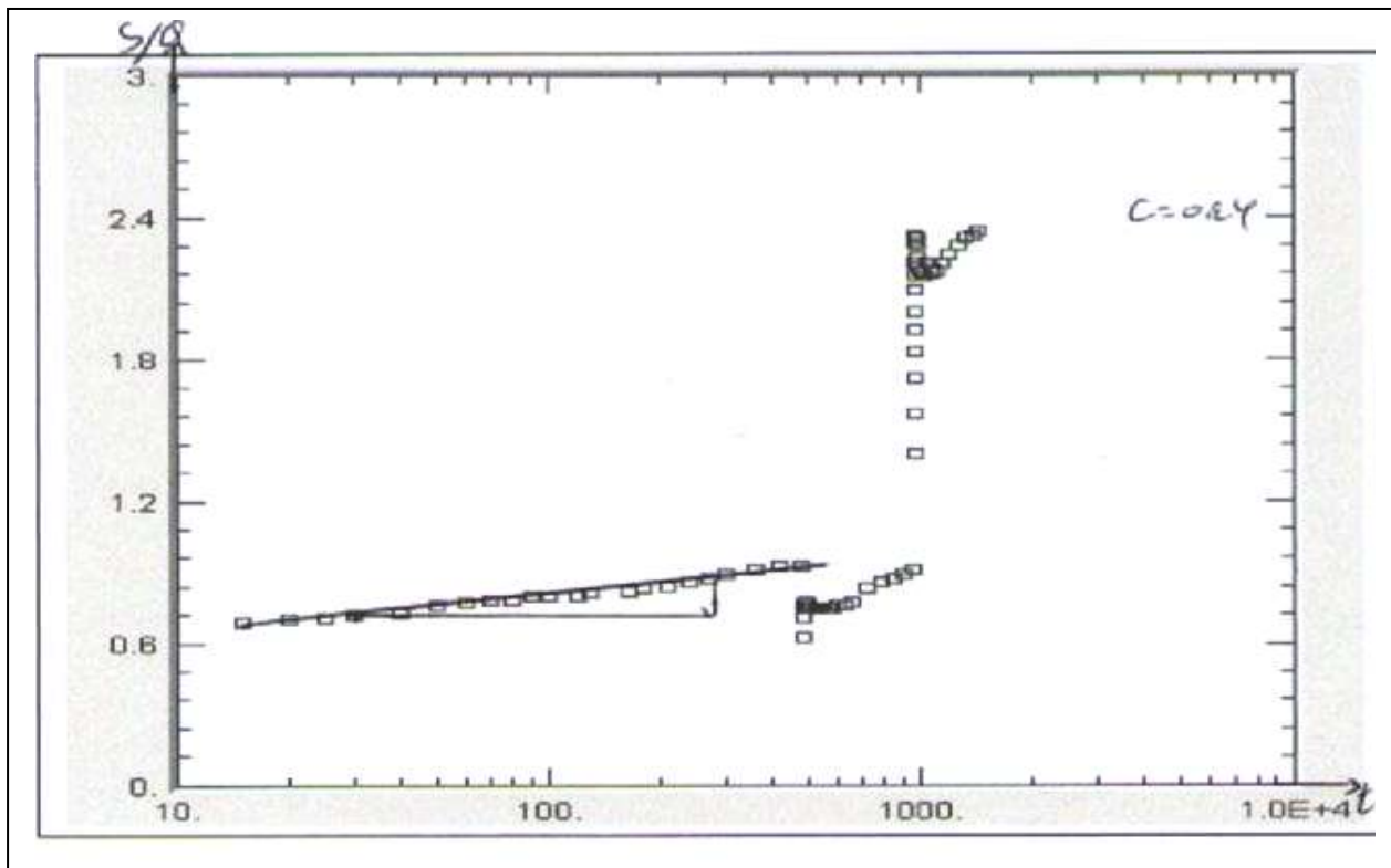
Figure III.15: courbe rabattement spécifique du forage F05 en fonction de temps (Pompage par palier de débits enchainés)
