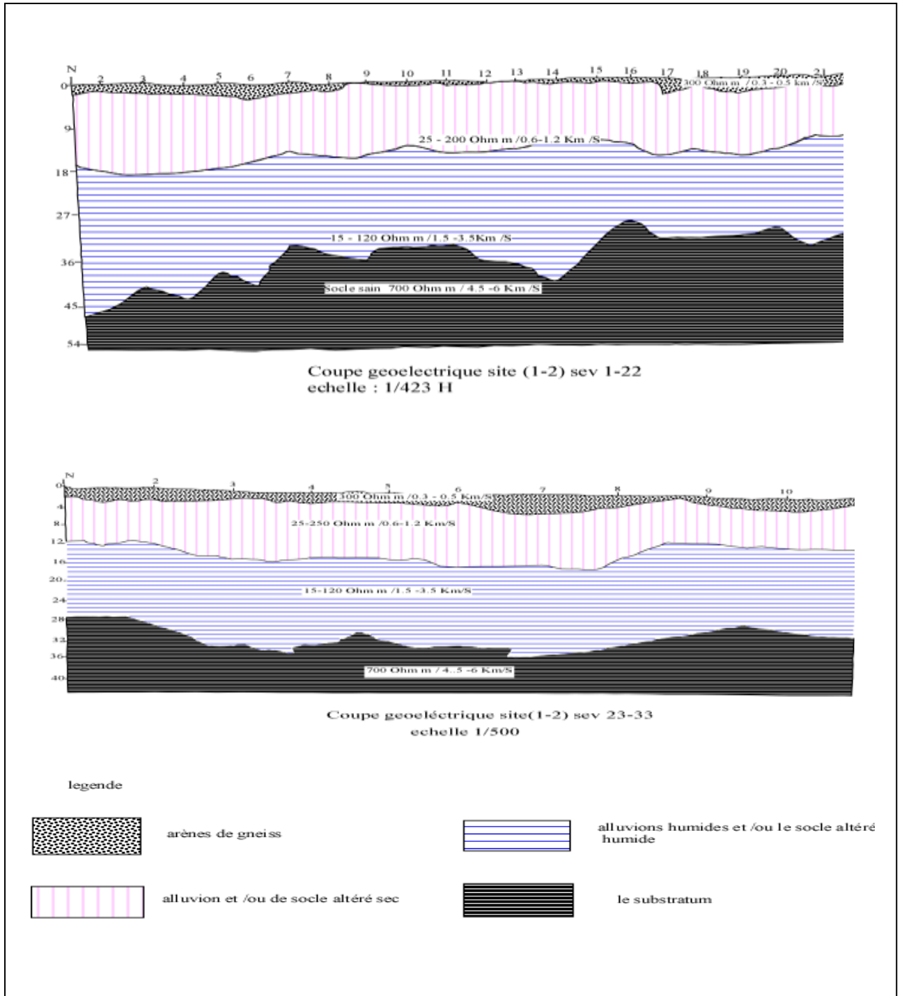
Figure I.20 : coupe géoélectrique site (1 -2) bureau d'étude DIALOG HYDRO-GEO-SERVICE(2001)
