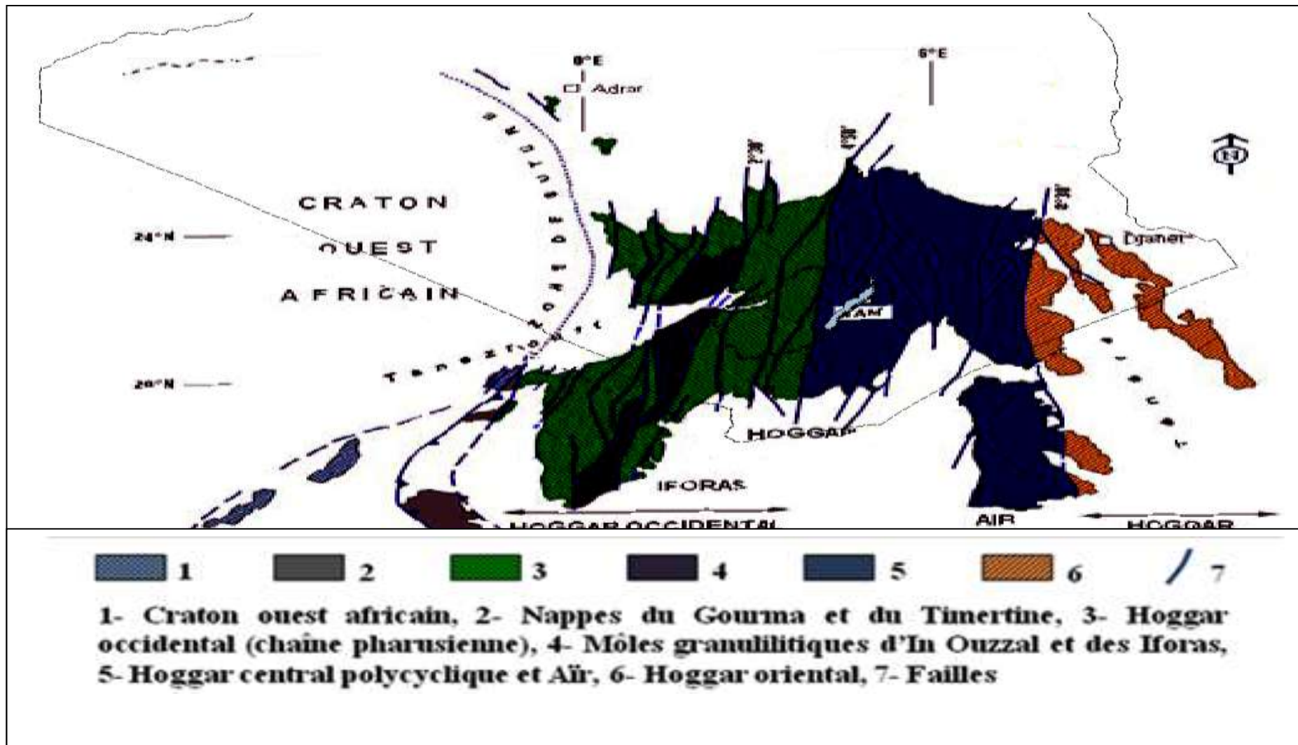
Figure I.4 : domaines structuraux du Bouclier Touareg (d'après Caby et al 1981 modifier par Boullier 1991)
