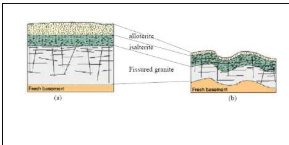
Figure III.2. (a) Profil d'altération monophasée sur granite (Wyns et al. 1999) et (b) profil d'altération polyphasée sur granite (Dewandel et al. 2006).
