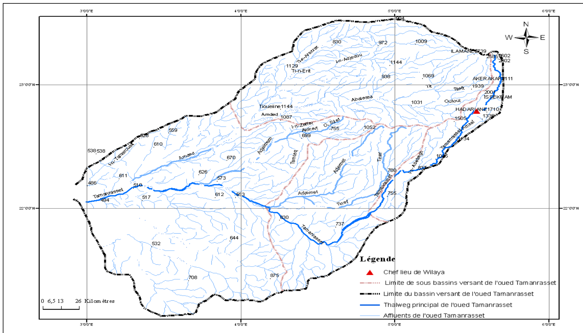
Figure II.1 : Le bassin versant de l'oued Tamarassset
