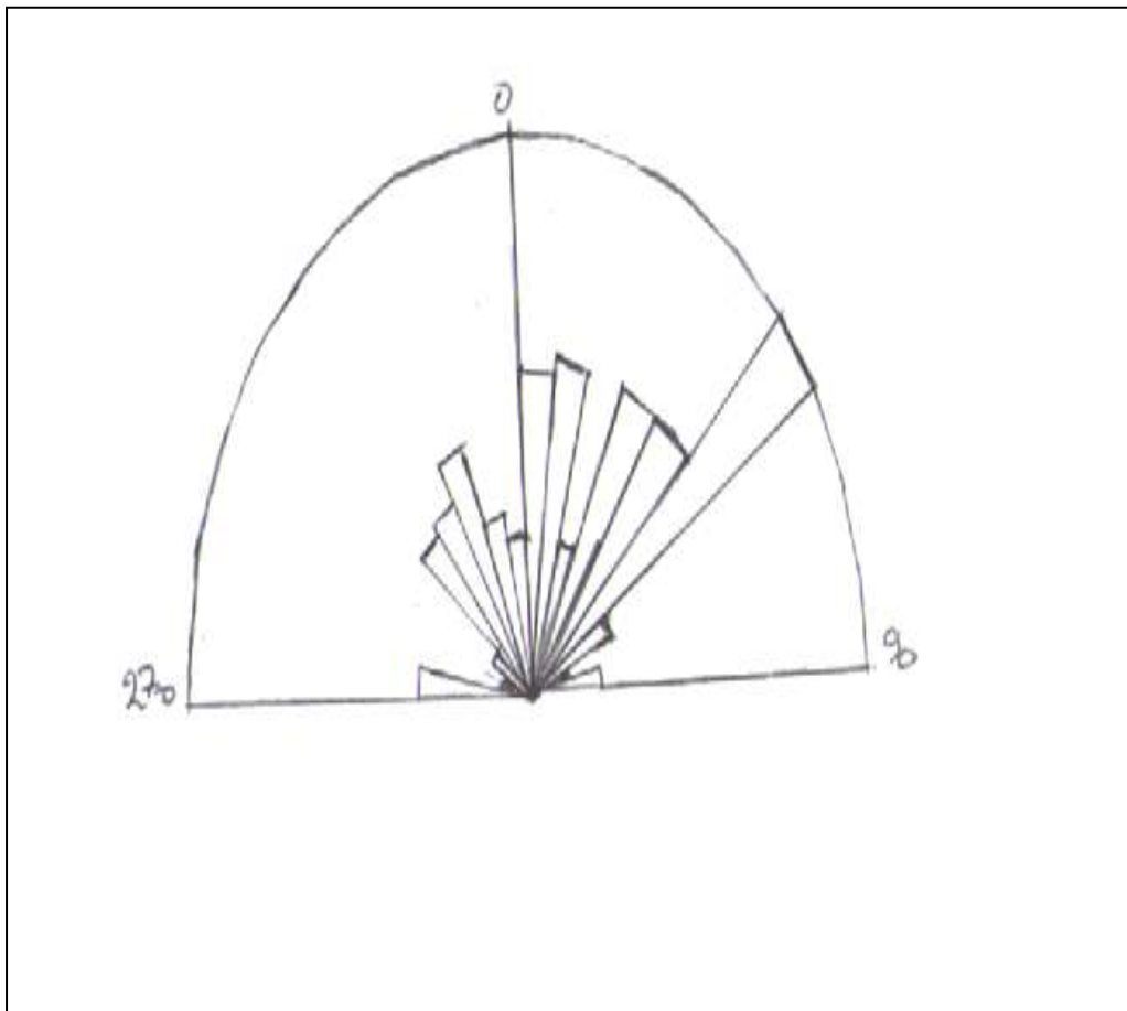
Figure I.15 : rosace directionnelle de la fracturation de socle de la zone d'étude Fréquence en nombre (N= 665).
