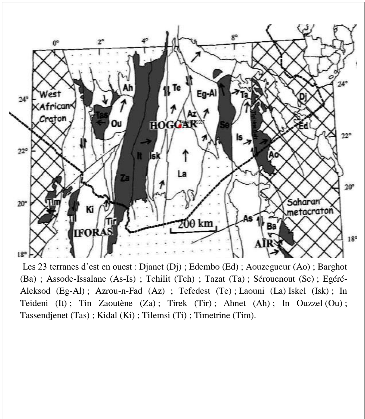
Figure I.5 : les différents terranes du Hoggar (Black et al 1994).
