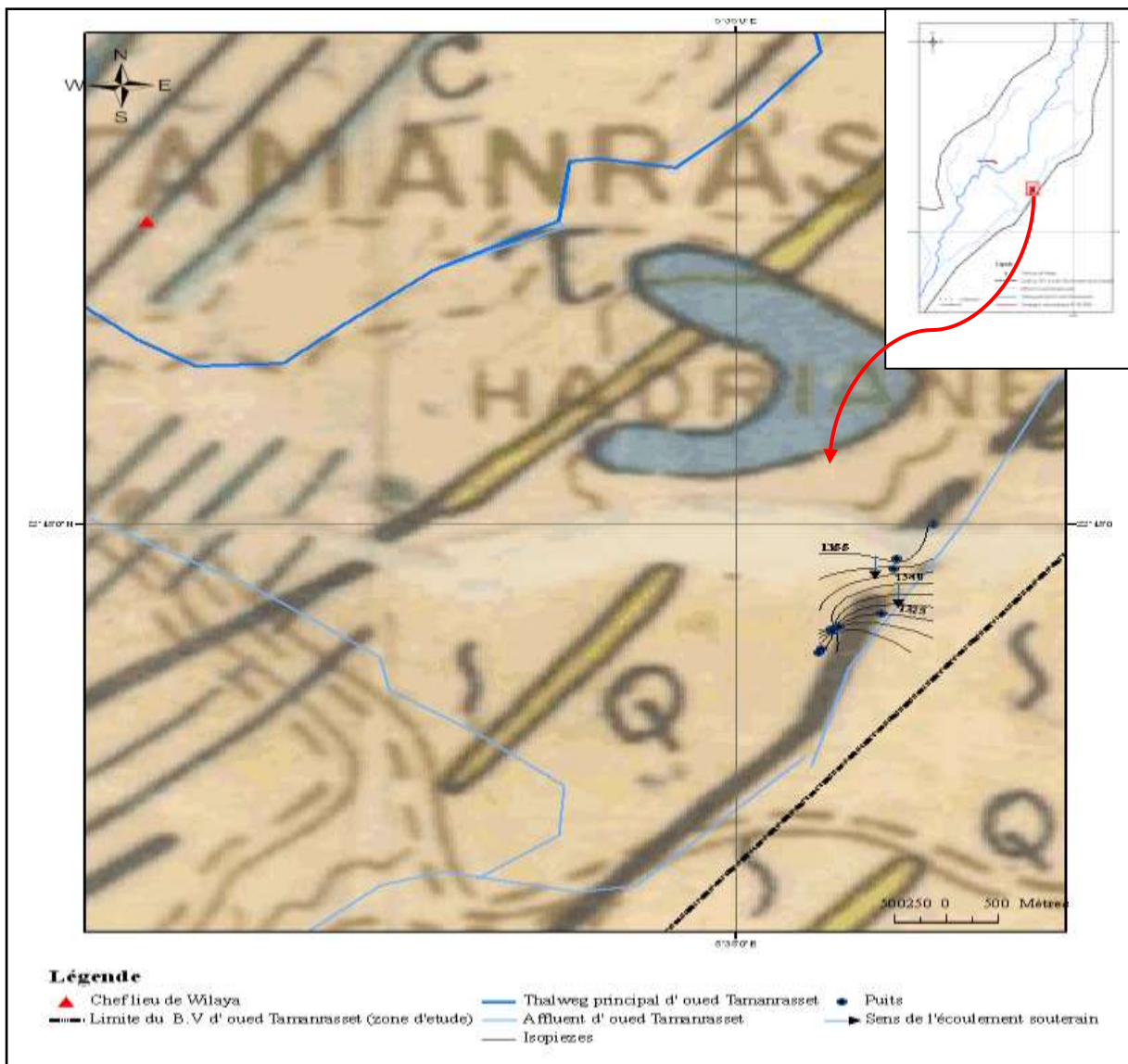
Figure III.9 : Carte piézométrique 01-04-2008 (Izerzi)
