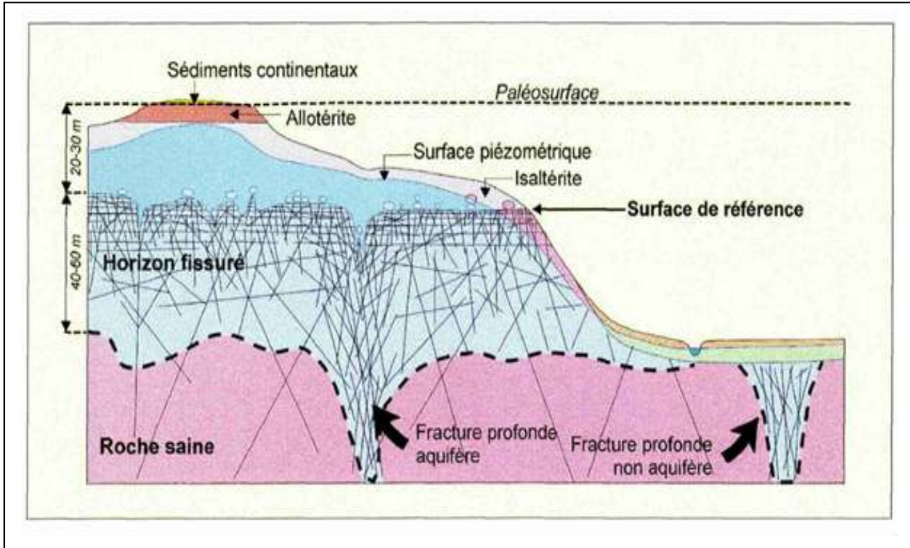
Figure III.1 : Schéma conceptuel de formation d'altération de roche de socle (Wyns 1999)
