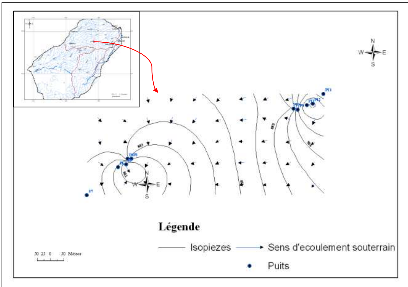
Figure III.12 : Carte piézométrique puits Ablessa 04-04- 2007
