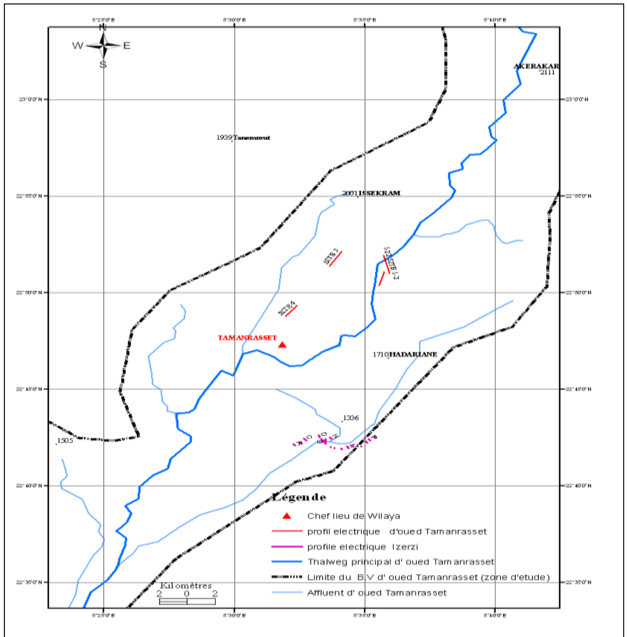
Figure I.19 : carte de situation des coupes géoélectriques
