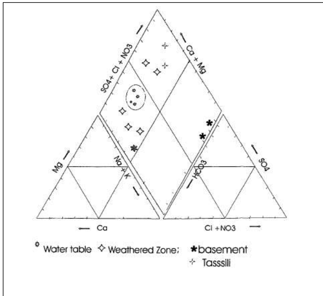
Figure IV .1 : diagramme de Piper de compositions chimique moyenne des eaux souterraines du Hoggar (O. SAIGHI J.L. MICHELOT, A. FILLY 2001)
