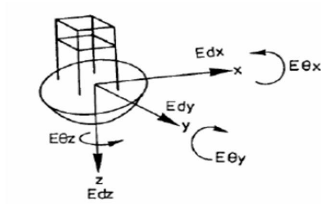
Fig 24: Composantes de l'action sismique
