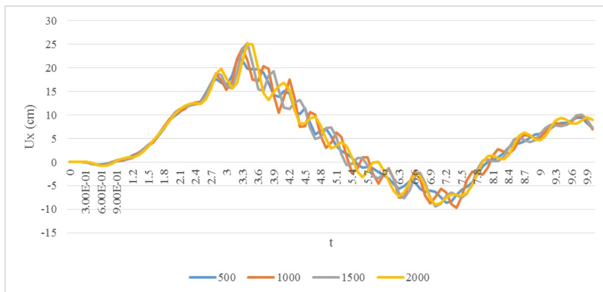
Fig V-28: influence de la densité du matériau granulaire contenu sur le déplacement latéral dans le sens d'application des excitations
