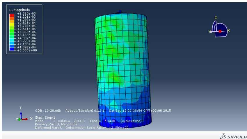
Fig V-8 : Les trois premiers modes de vibrations du modèle 2
