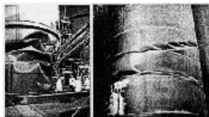
Fig I-8:Flambement d'une coque cylindrique sous compression axiale [9]
