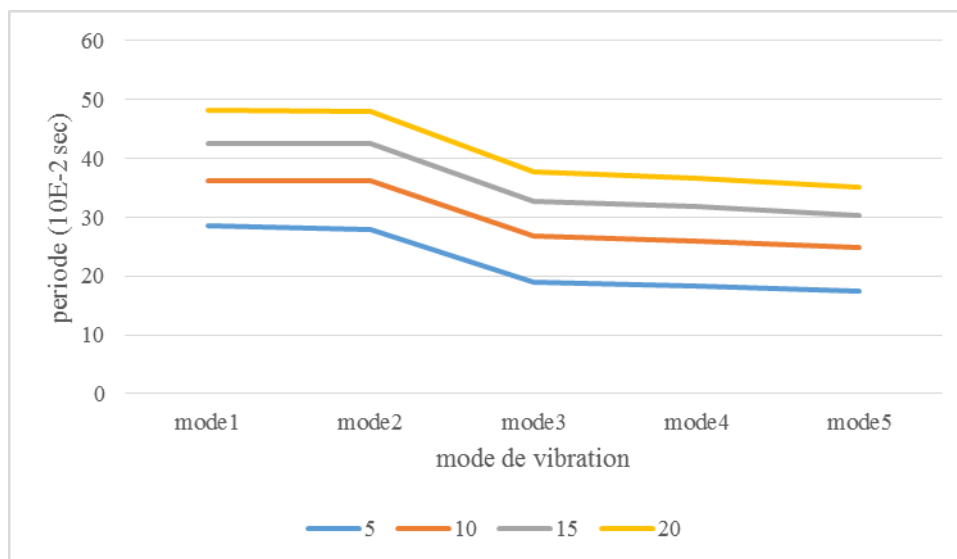
Fig V-27: variation des périodes naturelles pour les cinq premiers modes de vibrations du silo en fonction de la densité
