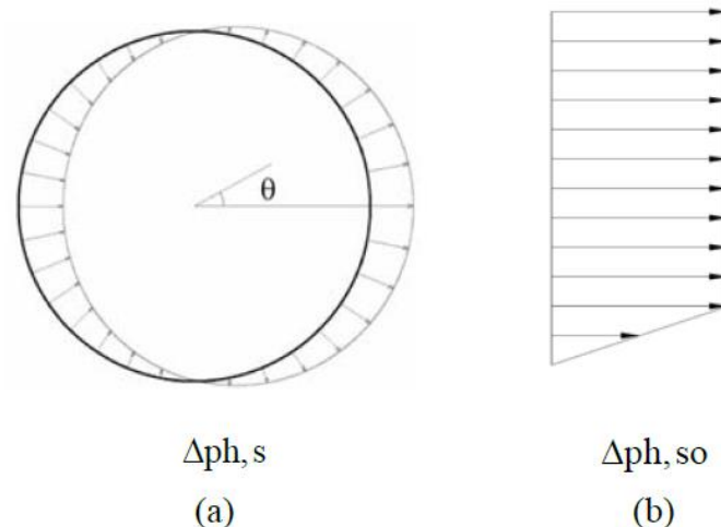
Figure IV-6 : (a) La distribution de \Delta ph,so dans la section du silo, (b) La répartition des \Delta ph,s sur la hauteur du silo [33].
