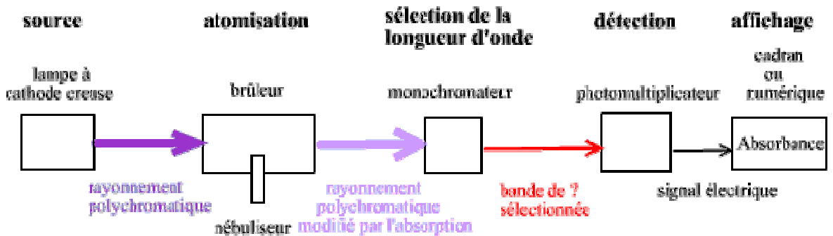
Schéma descriptif de la spectroscopie d'absorption atomique
