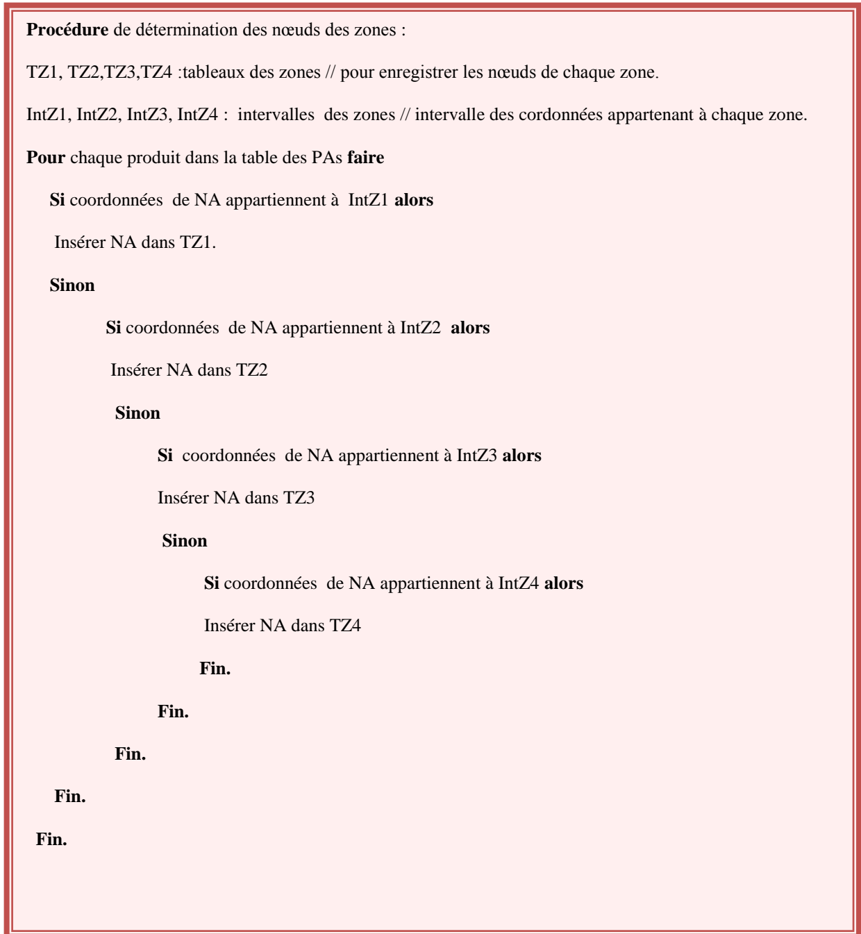
Figure V-14 pseudo code de détermination des nœuds de chaque zone.
