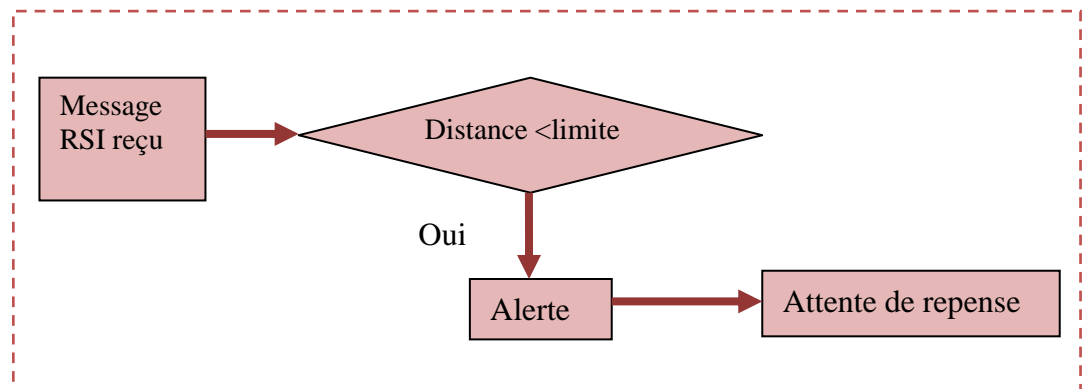
Figure V-17 diagramme de surveillance de la distance.
